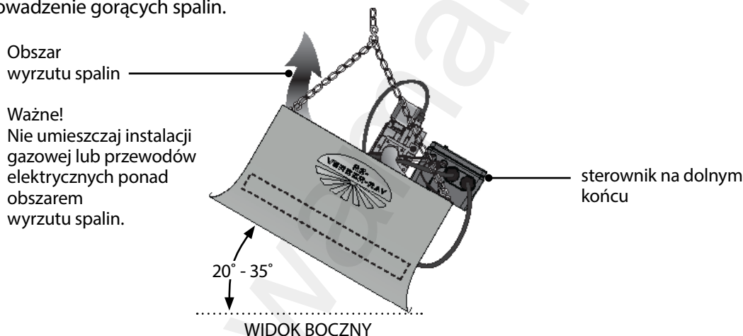
Rys. 2.4 • Odprowadzenie gorących spalin.
