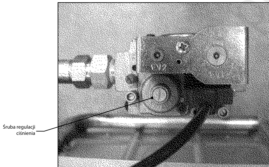
Rys. 4.5 · Śruba regulacji ciśnienia zaworu gazowego.
