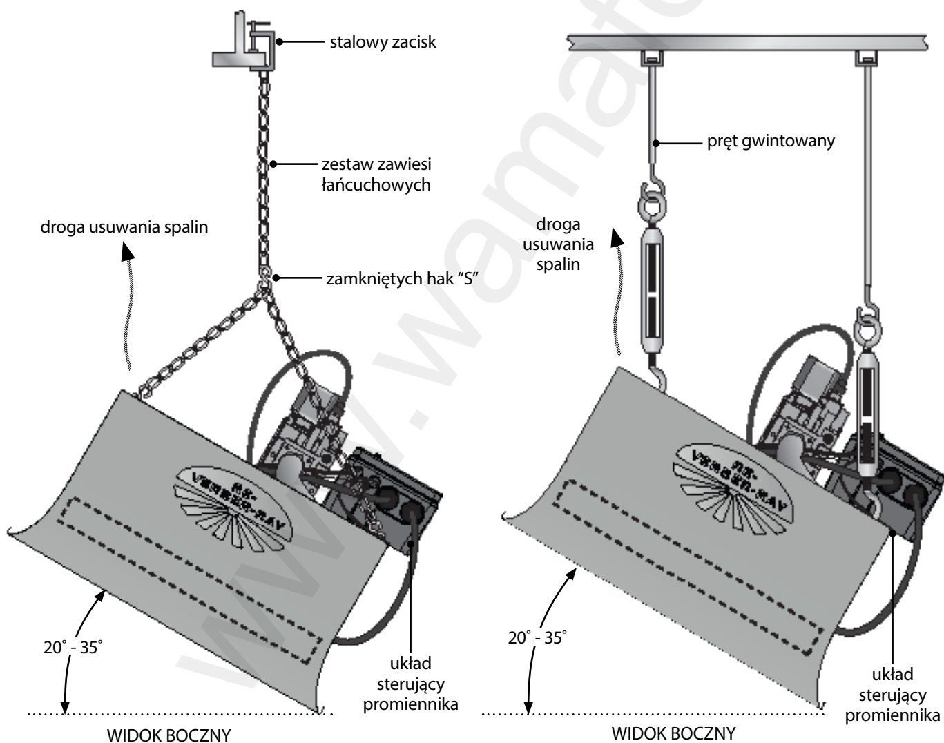
Rys. 2.3 • Przykładowe sposoby montażu
