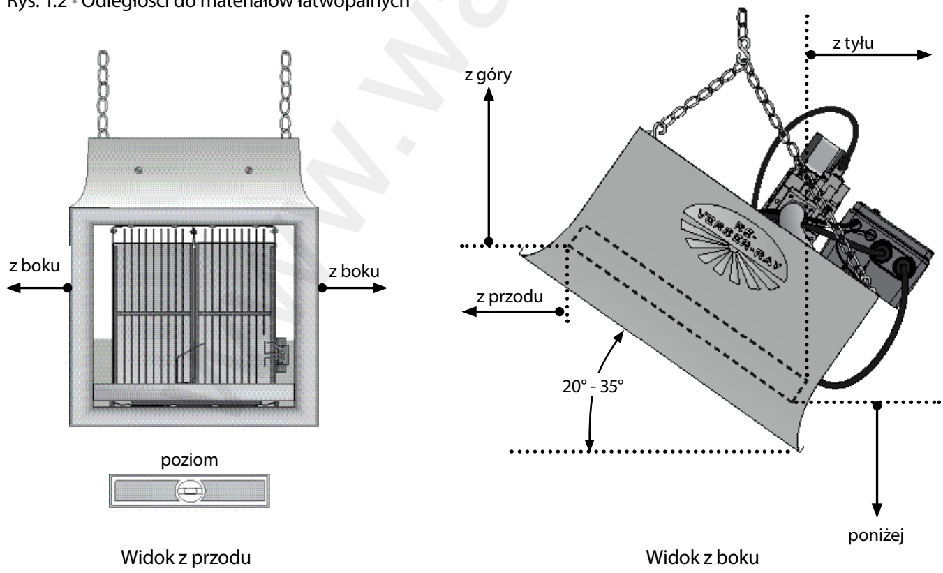
Rys. 1.2 • Odległości do materiałów łatwopalnych
