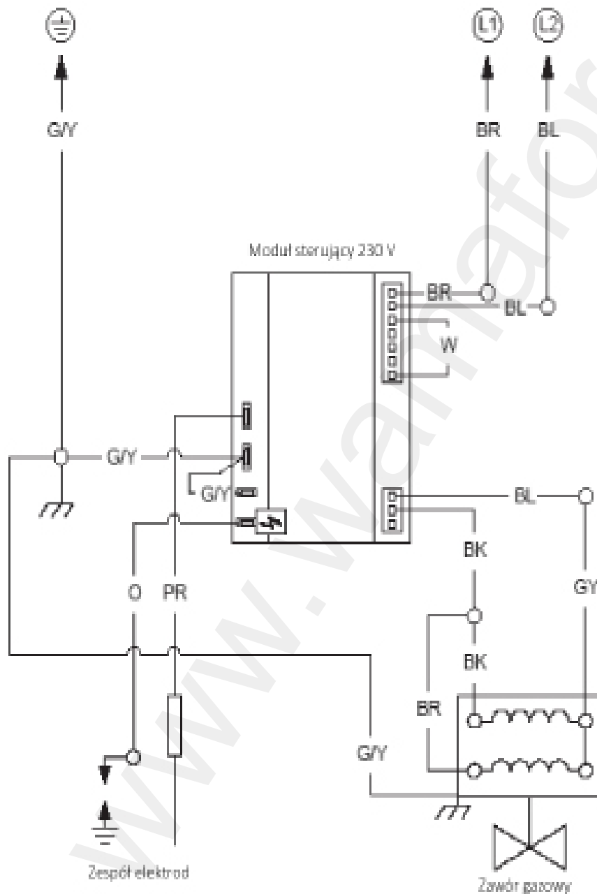
Rys. 2.5 Schemat połączeń płytki elektronicznej 230 V do promiennika DR.
